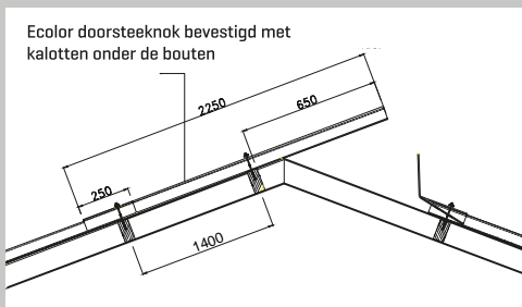
Ecolor doorsteeknok voorzien van kalotten onder de bouten
